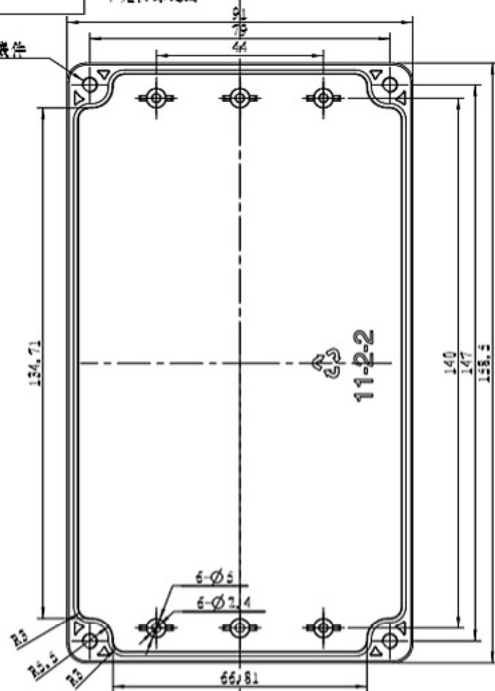
下壳内部视图
