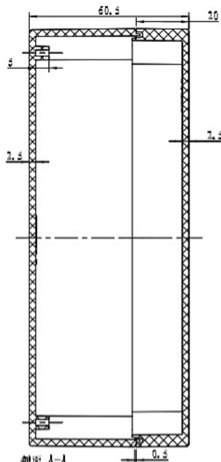
剖面 A-A
