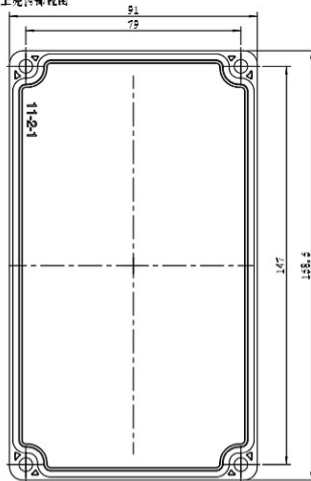
上壳内部视图
