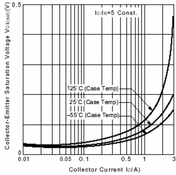
Fig.4 V_{ce(sat)}-I_c
