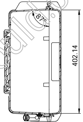
剖面 A-A
