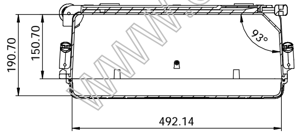
剖面 C-C
