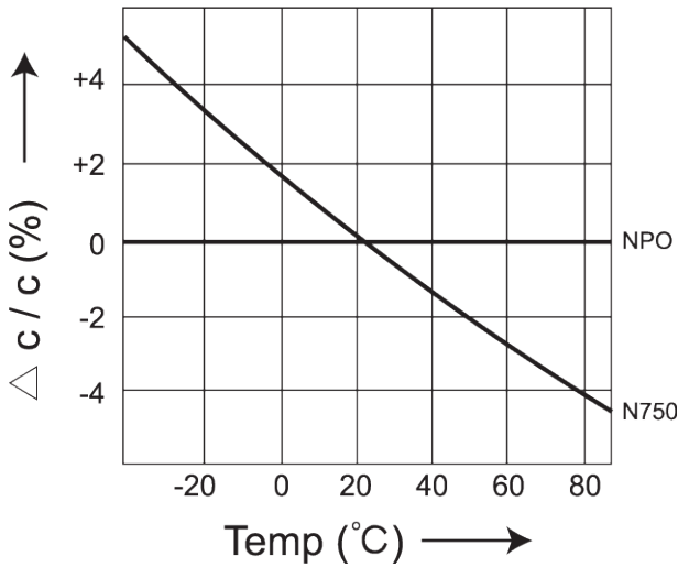
Fig. 1A (T. C. PPM/°C) NPO
