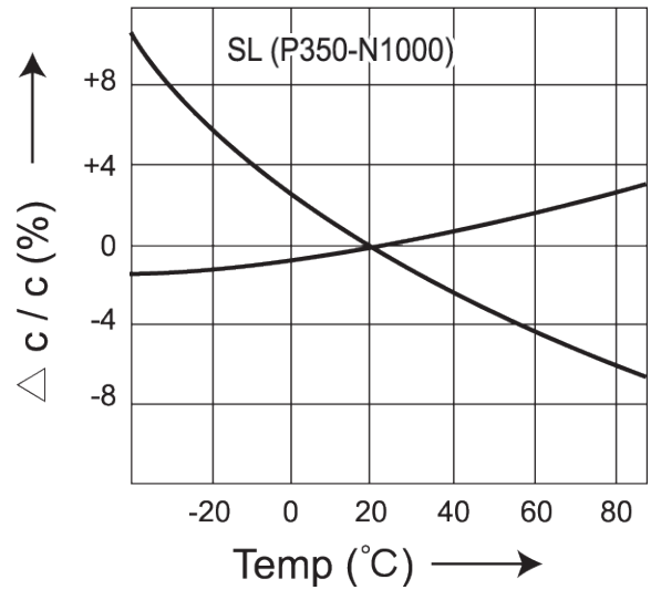
Fig. 1B SL (P350-N1000)
