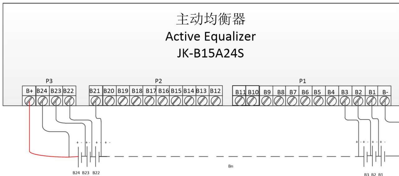
JK-B15A24S 接线图
