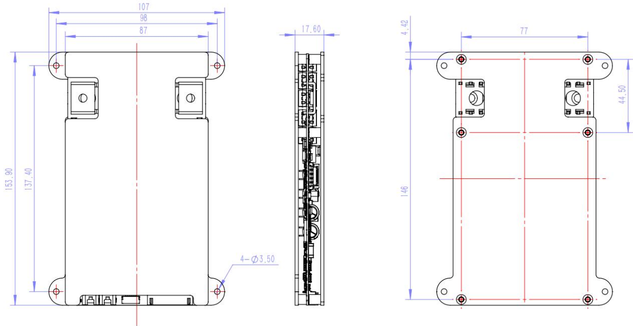
JK-B1A8S-10PS 外形尺寸
