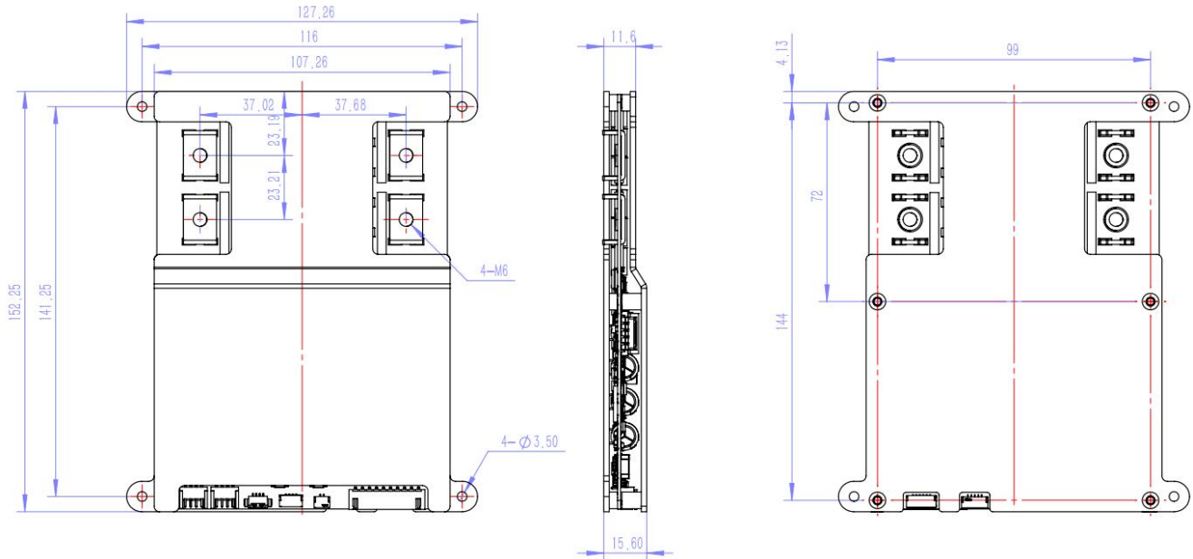
JK-BxA8S-20PS 外形尺寸
