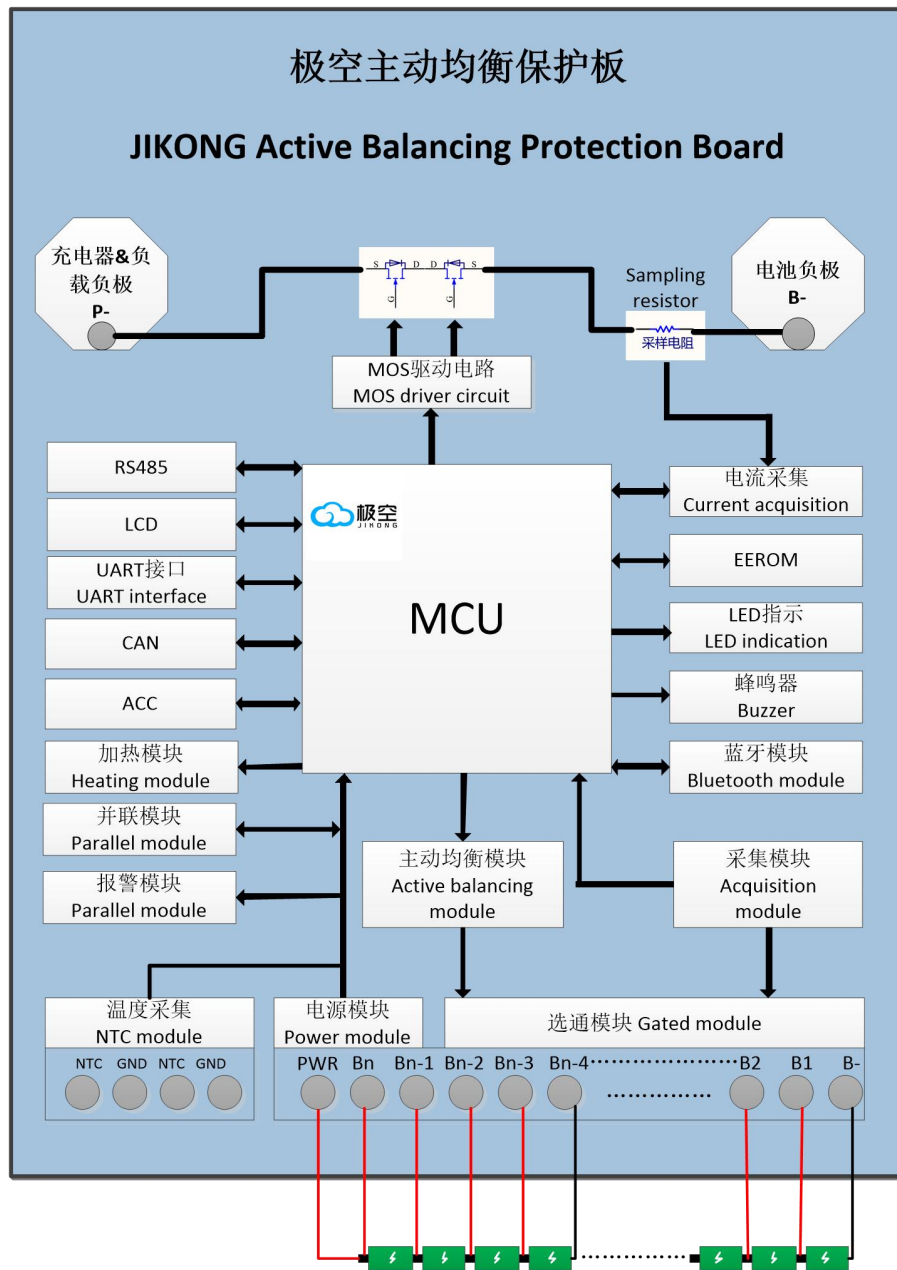
JK-BxA8S-20PS 结构框图
