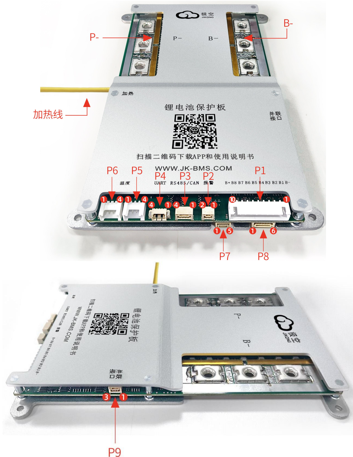
JK-B2A8S-30PS 连接器示意图
