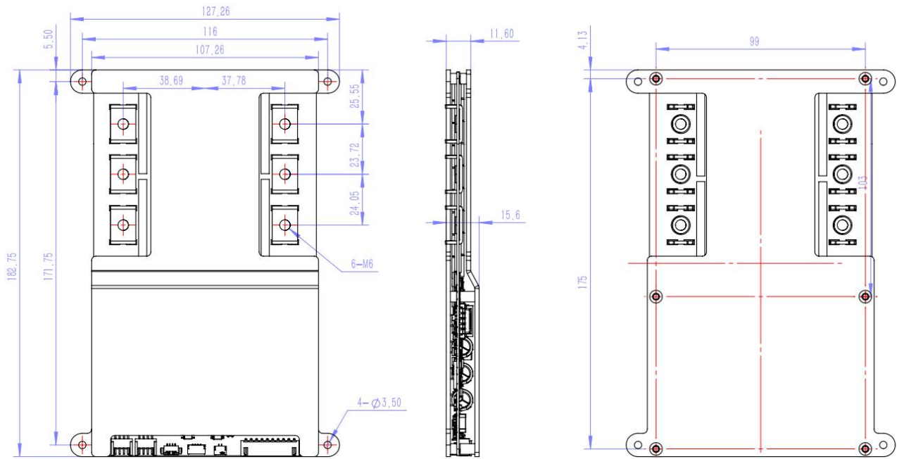
JK-B2A8S-30PS 外形尺寸
