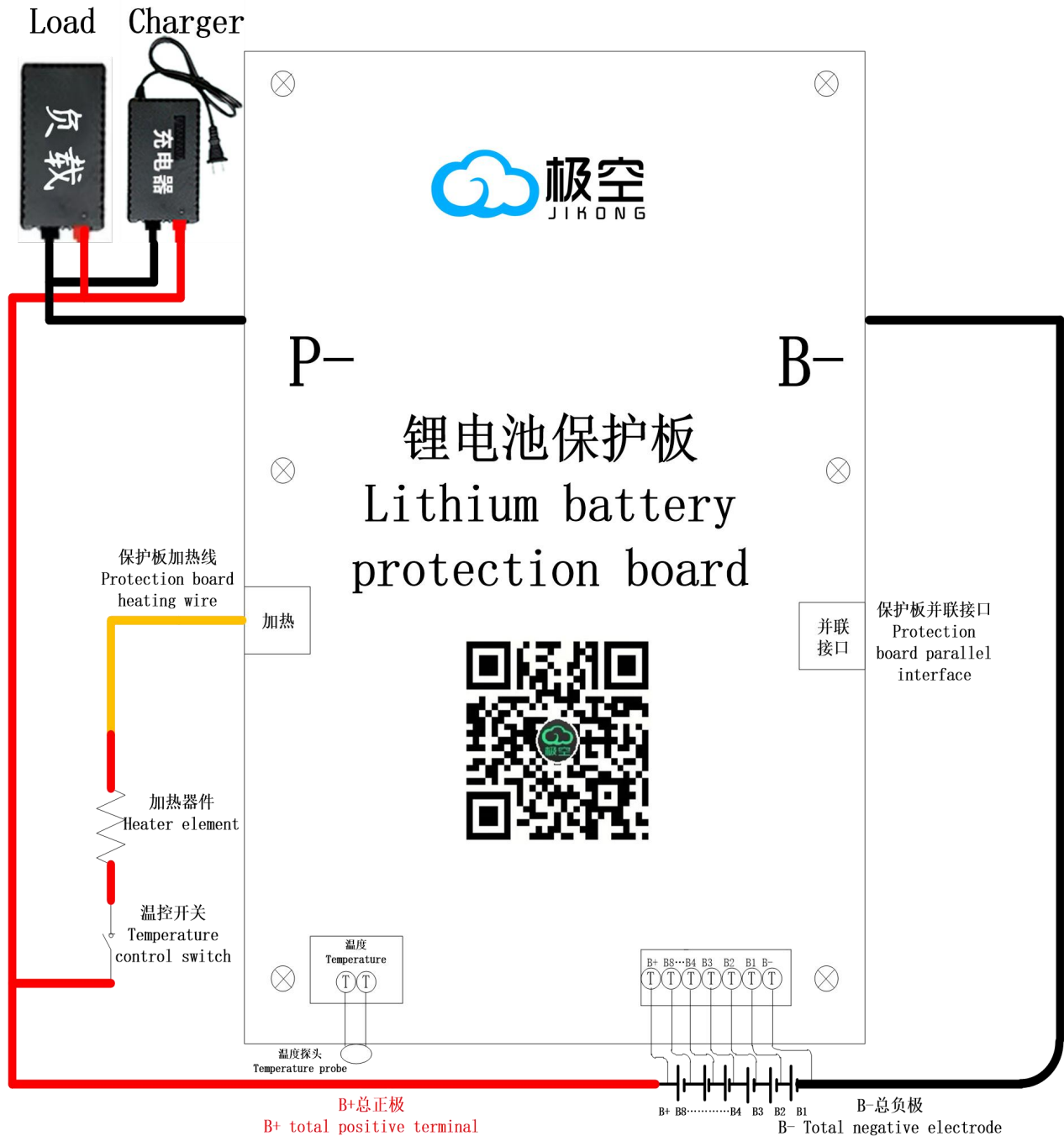
JK-B2A8S-30PS接线图
