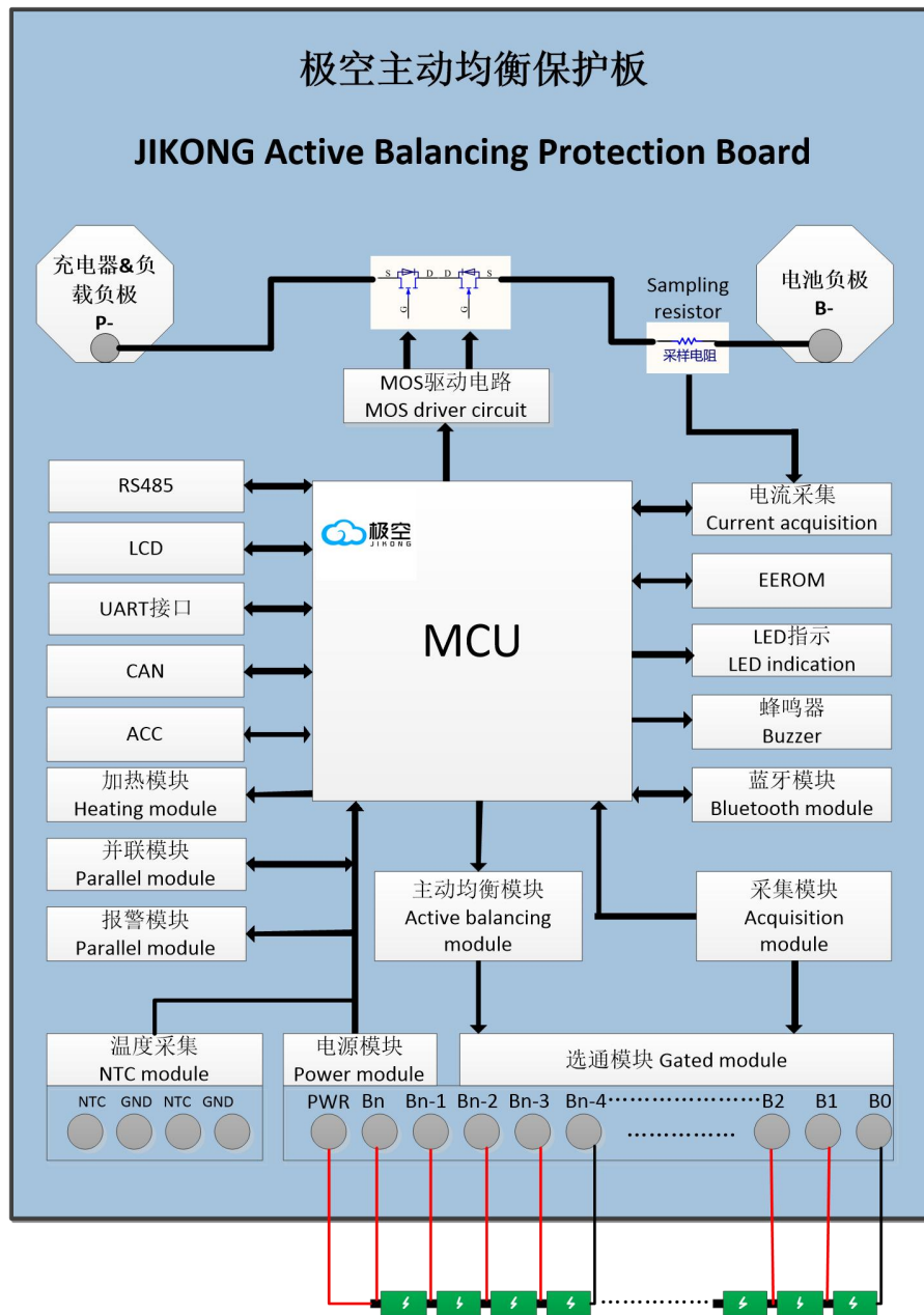
JK-B2A8S-30PS 结构框图
