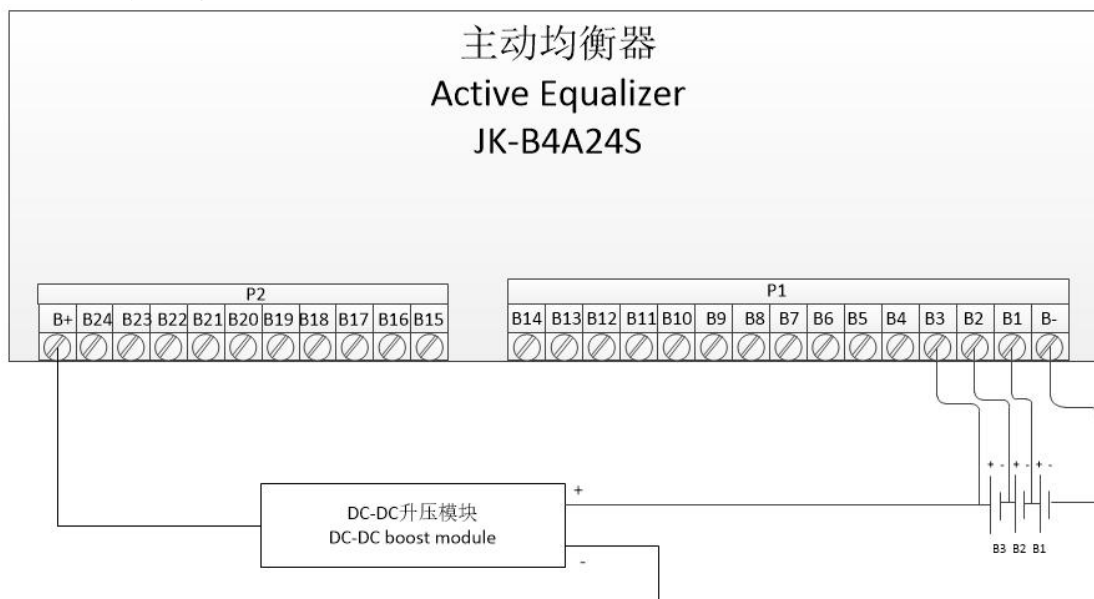
配合升压模块接线图
