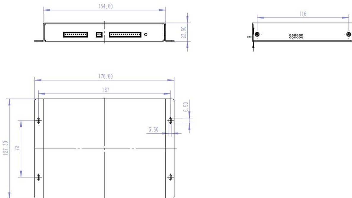
JK-B4A24S 外形尺寸
