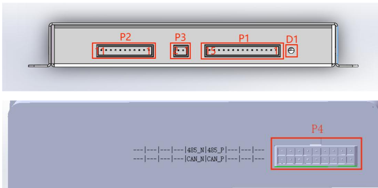
JK-B4A24S 连接器示意图
