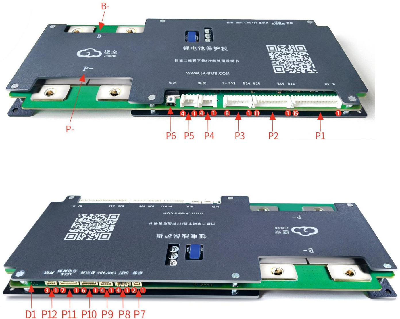
JK-BD6A32S-10P连接器示意图
