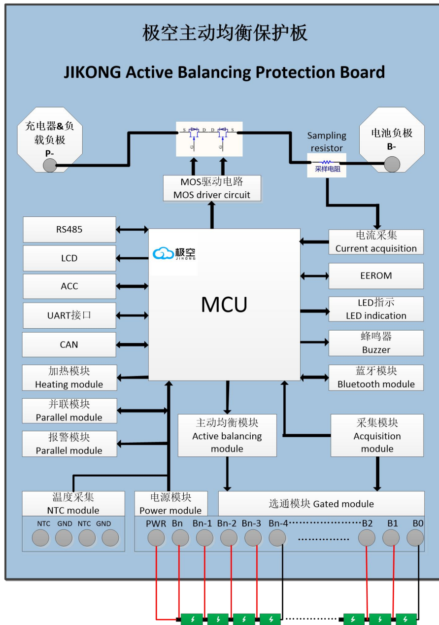
JK-BD6A32S-10P/15P结构框图
