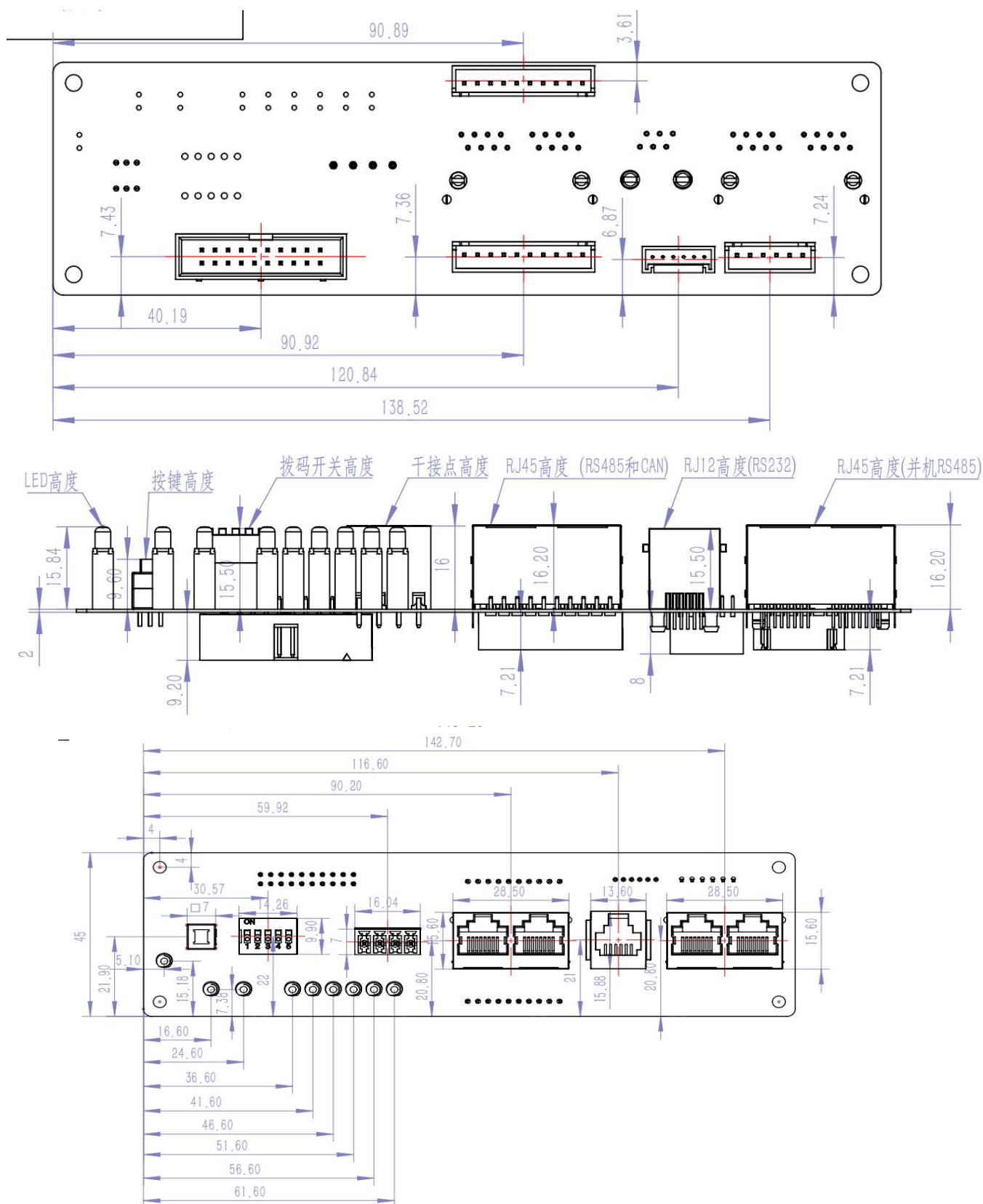
接口板 外形尺寸
