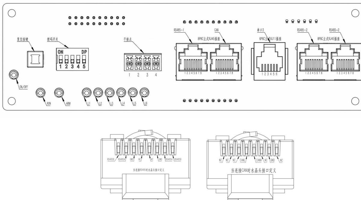
接口板接口示意图 Interface board interface diagram
