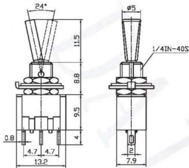
外型图 (Outline Drawing)
