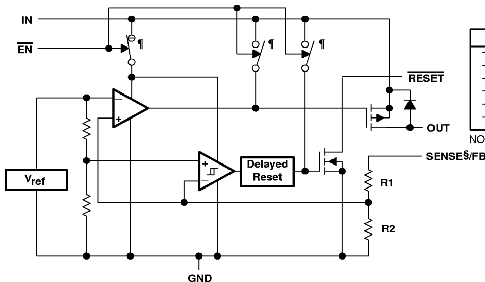
RESISTOR DIVIDER OPTIONS
