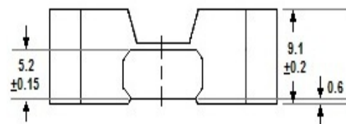
EFD25/13/9 полусердечник
