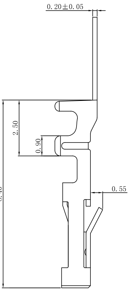
SEC:A-A
