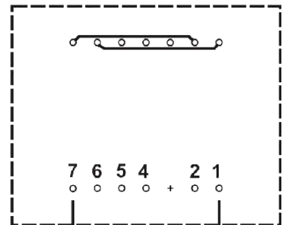
7 6 5 4 2 1 Первичная обмотка
