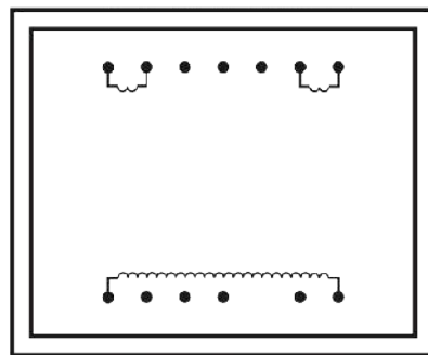
7 6 5 4 2 1 Первичная обмотка
